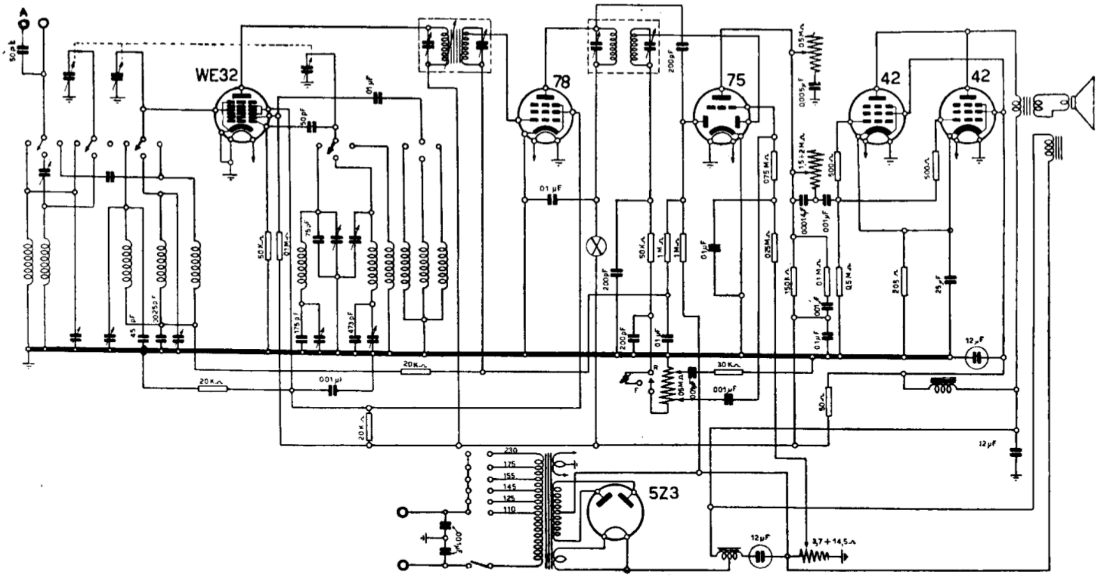
MAGNADYNE RADIO. — Mod. « SV 12, SV 14, SV 17, SV 112, SV 114 e SV 117 ». — Media frequenza: 362,5 kHz. Produzione: 1936.
